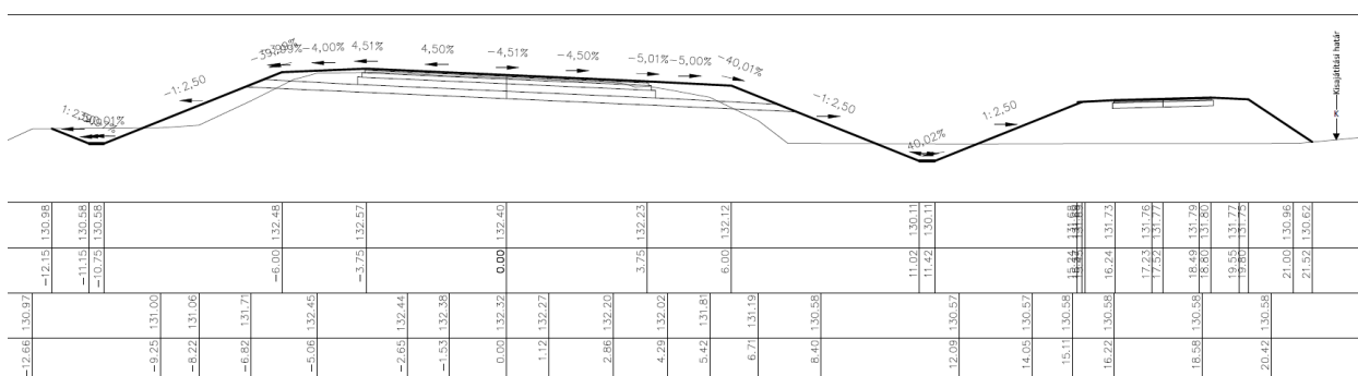
4. ábra: A főút és kerékpárút jellemző keresztmetszete 70+684 km szelvényénél Kelevízen
