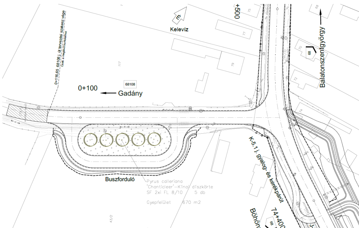
2. ábra: Új buszforduló terve Kelevízen
