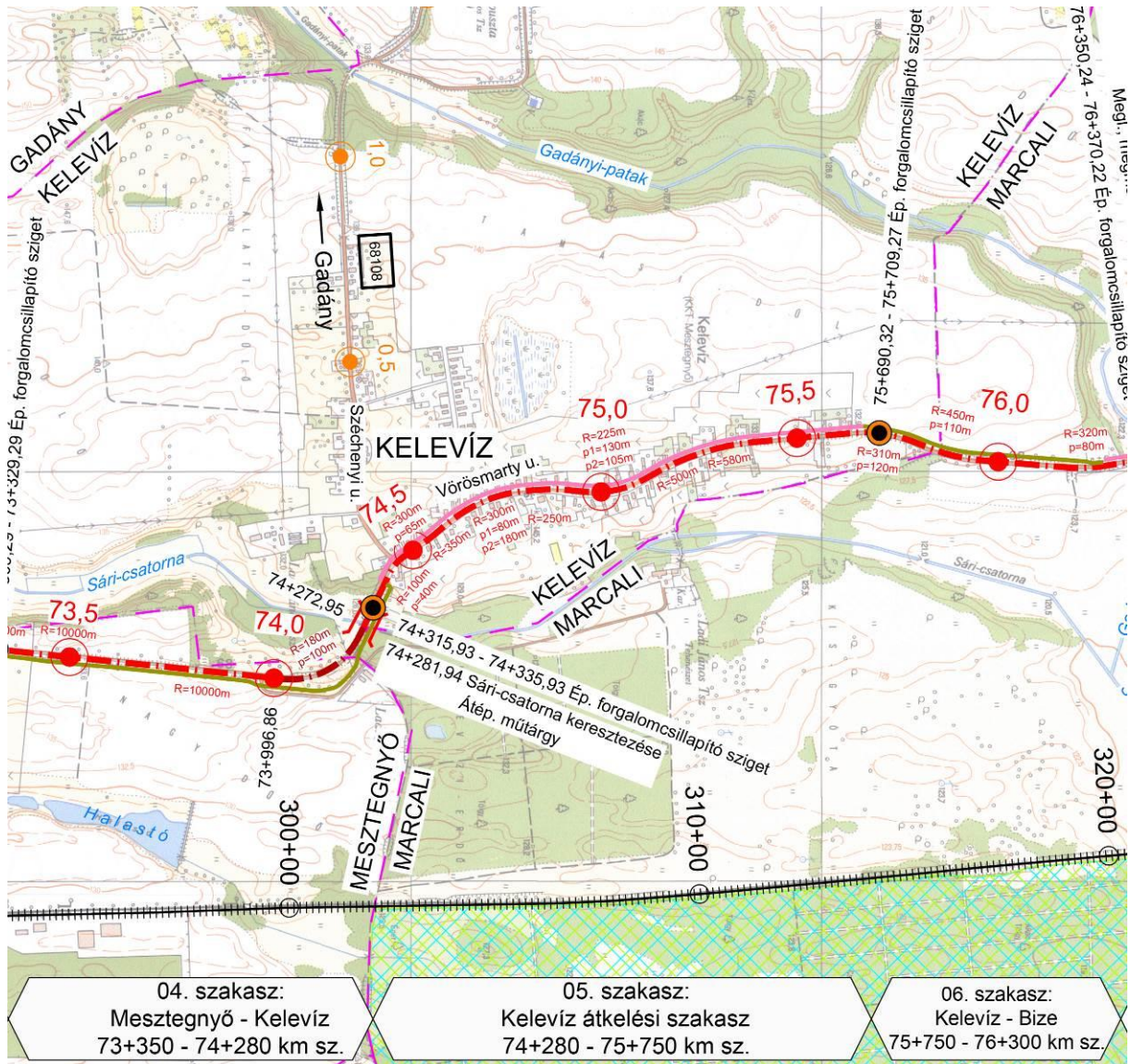
1. ábra: Útépítési terv átnézeti helyszínrajza (forrás: Pannonway Építő Kft.)
