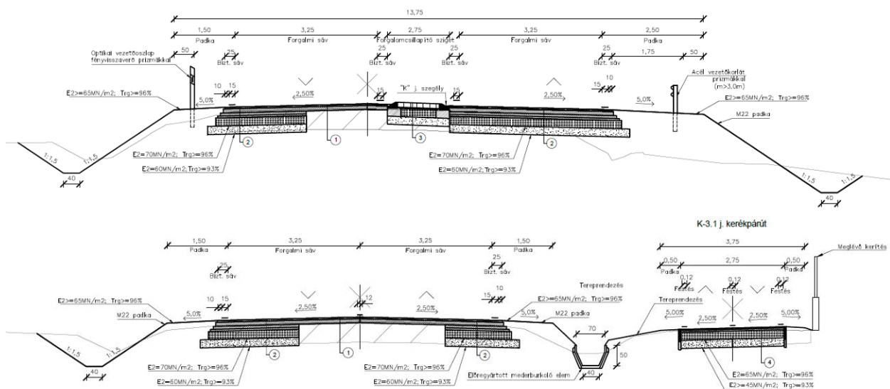
3. ábra: Forgalomcsillapító szigetek típuskeresztmetszetei
