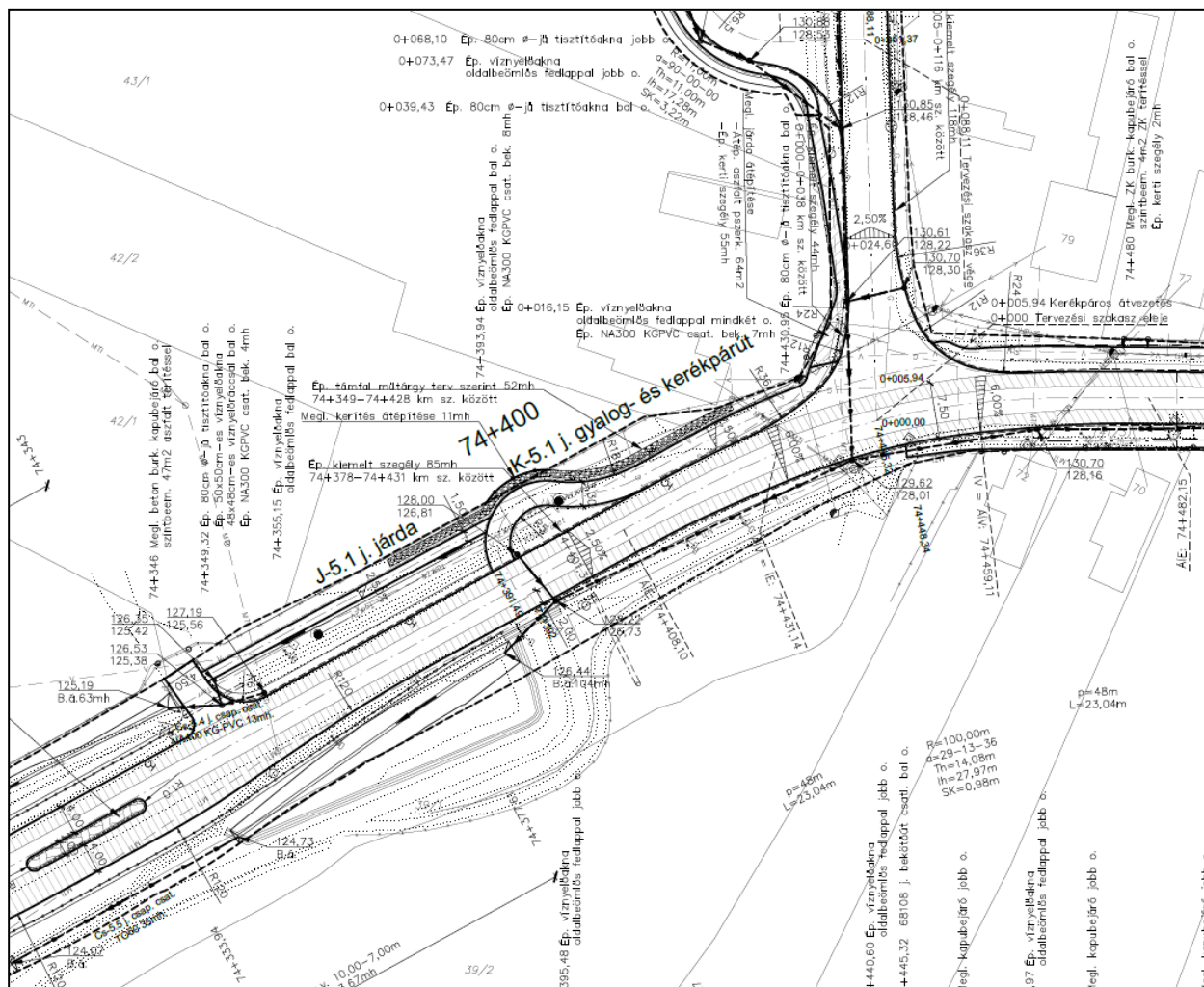
74+270 – 74+900 km sz. helyszínrajz részlete
